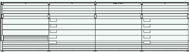
LS 168 24 x 8,1 x 7,8 m 168 sittplatser, 4 sektioner
