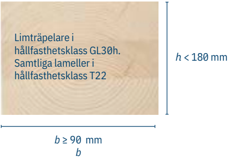
Homogen limträbalk
